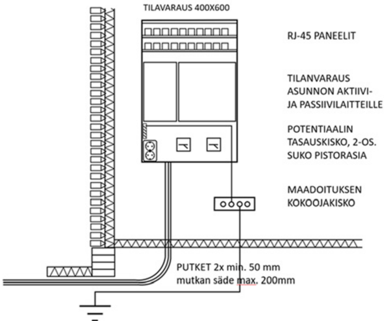
Kuva 1: Kaapelin tuonti kiinteistöön.
